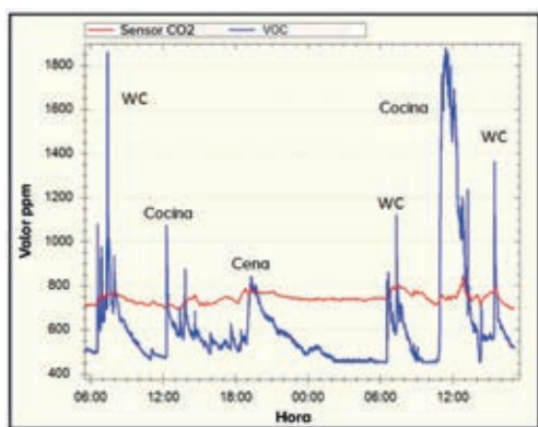
El diagrama muestra la comparación del sensor de CO 2 y VOC
