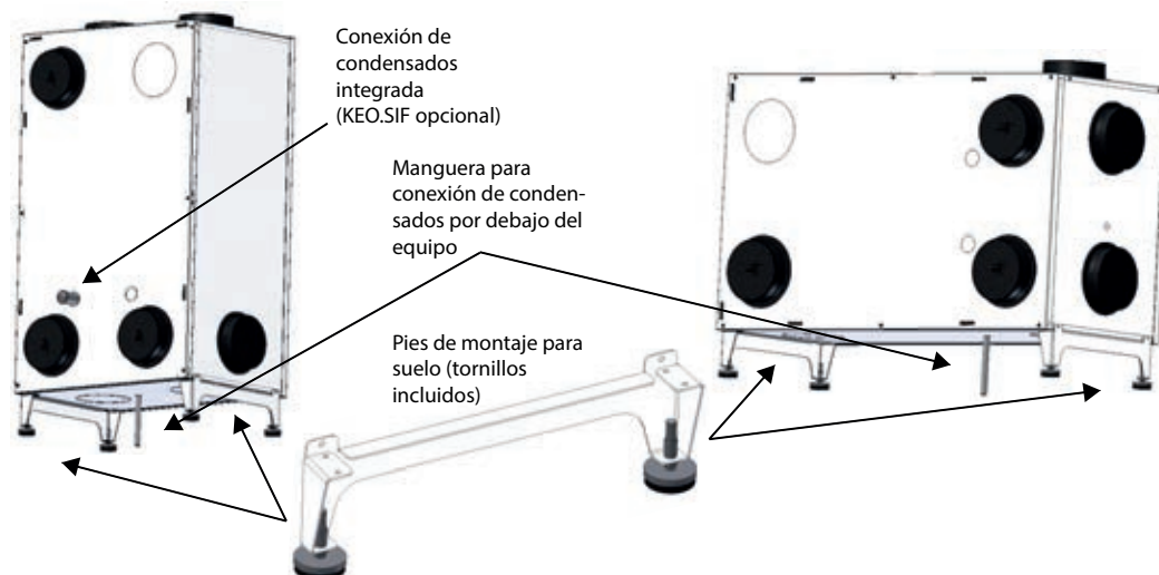
Montaje en suelo vertical
