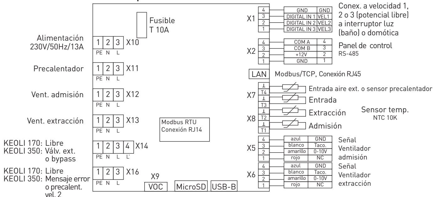
Esquema eléctrico Keoli
