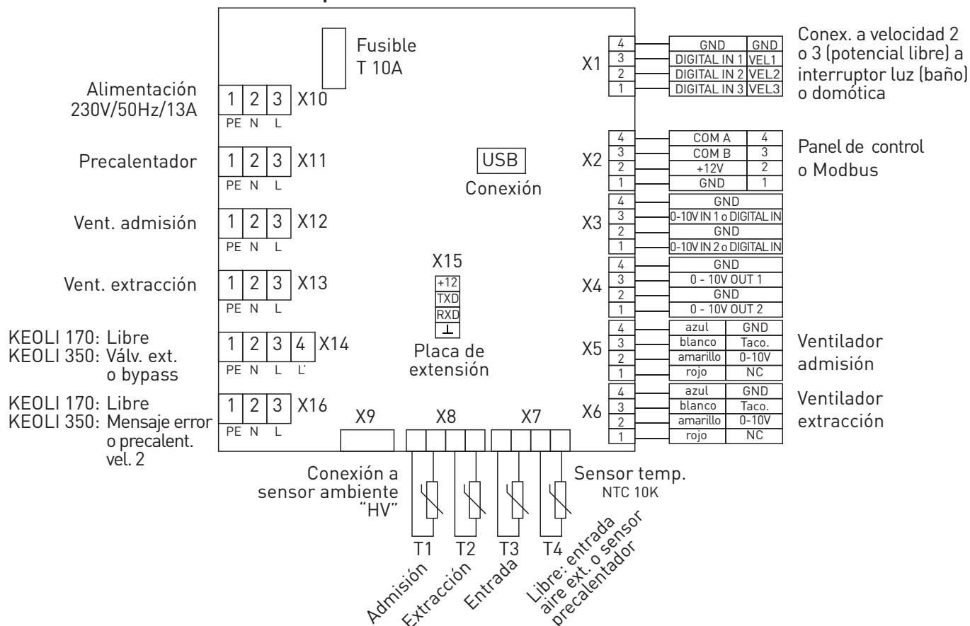
Esquema eléctrico Keoli
