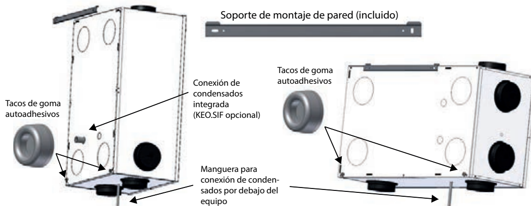
Montaje en pared vertical
