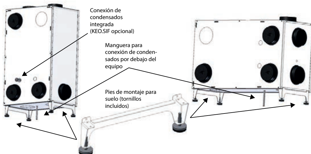
Montaje en suelo vertical
